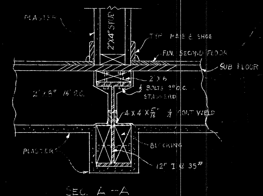
SEC. A-A
